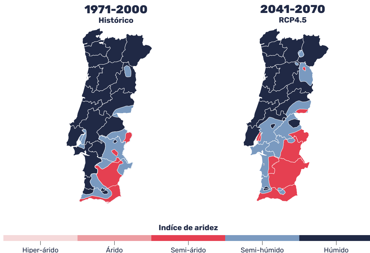
Figura 5. Projeções de evolução do índice de aridez em Portugal continental para um cenário intermédio de emissões de GEE.
